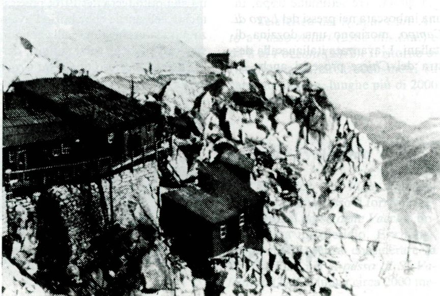
CIMA CARÈ ALTO: STAZIONE DI ARRIVO DELLA TELEFERICA DAL RIFUGIO CARÈ ALTO (LA PIÙ ALTA DI TUTTO IL FRONTE ALPINO (Foto: H.v. Lichem - Cortesia: ing. Dante Ongari).
