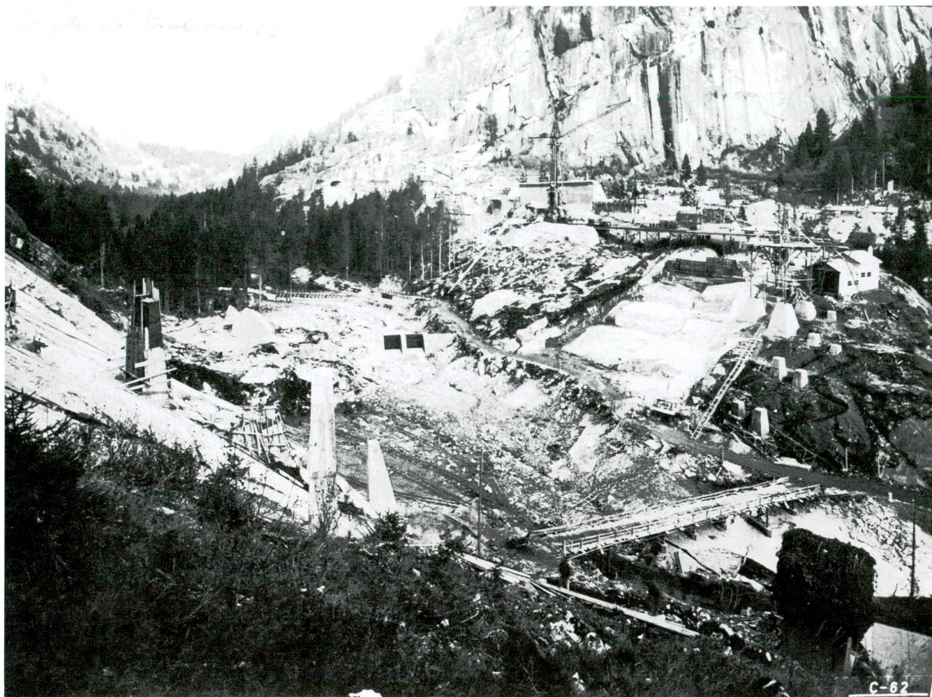
VAL DI DAONE - ANNO 1953: LAVORI DI COSTRUZIONE DELLA DIGA DEL BACINO IDROELETTRICO DI «BOAZZO» (Cortesia: Livio Losa).
