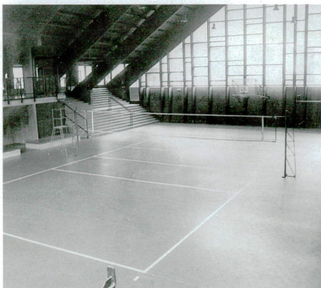
Creto - Pavimentazione palestra (foto Ruggero Rota).
