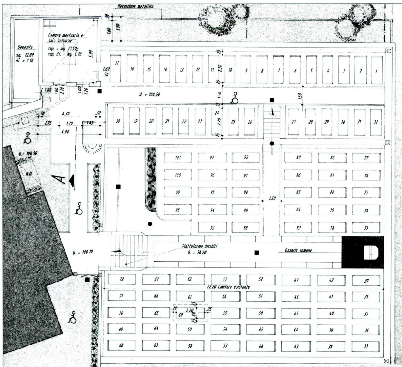
Pianta del Cimitero secondo nuovo progetto (dott. arch. Aldo Mazzoli, Pinzolo).
