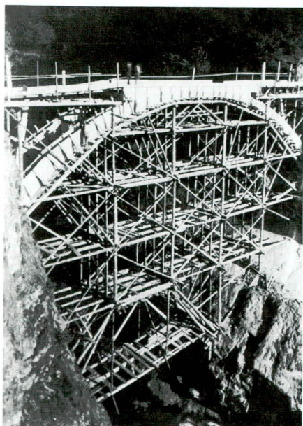
Sul retro delle foto: PONTE SUL FIUME CHIESE NEL COMUNE CATASTALE DELLE FRAZIONI DI BERSONE E FIRMINO IN VALLE GIUDICARIE (PROV. DI TRENTO) - IN FASE DI COSTRUZIONE E FINITO (Fotografia Arturo Ghirardini, Tione - Trentino).
