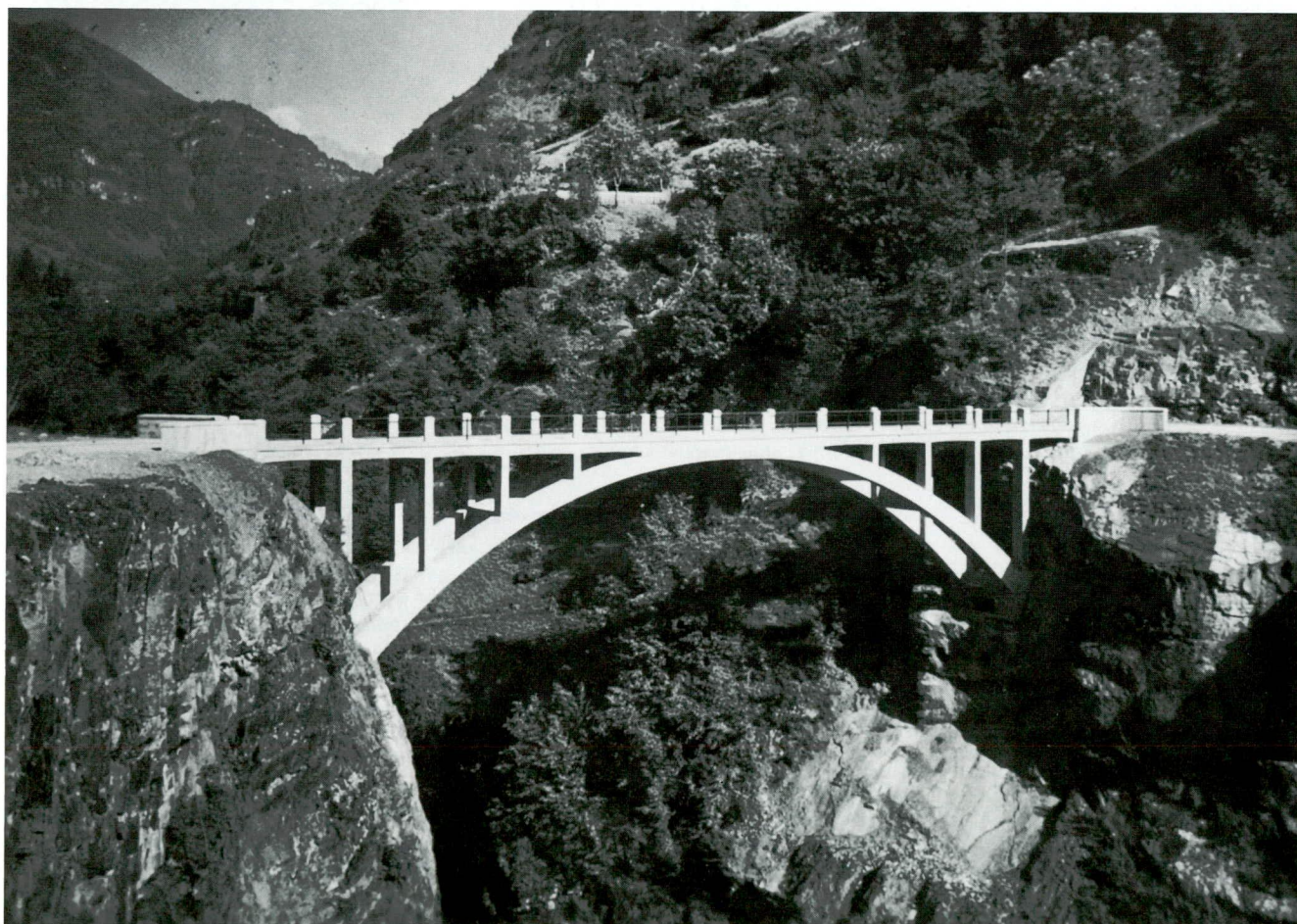
Sul retro delle foto: PONTE SUL FIUME CHIESE NEL COMUNE CATASTALE DELLE FRAZIONI DI BERSONE E FIRMINO IN VALLE GIUDICARIE (PROV. DI TRENTO) - IN FASE DI COSTRUZIONE E FINITO (Fotografia Arturo Ghirardini, Tione - Trentino).
