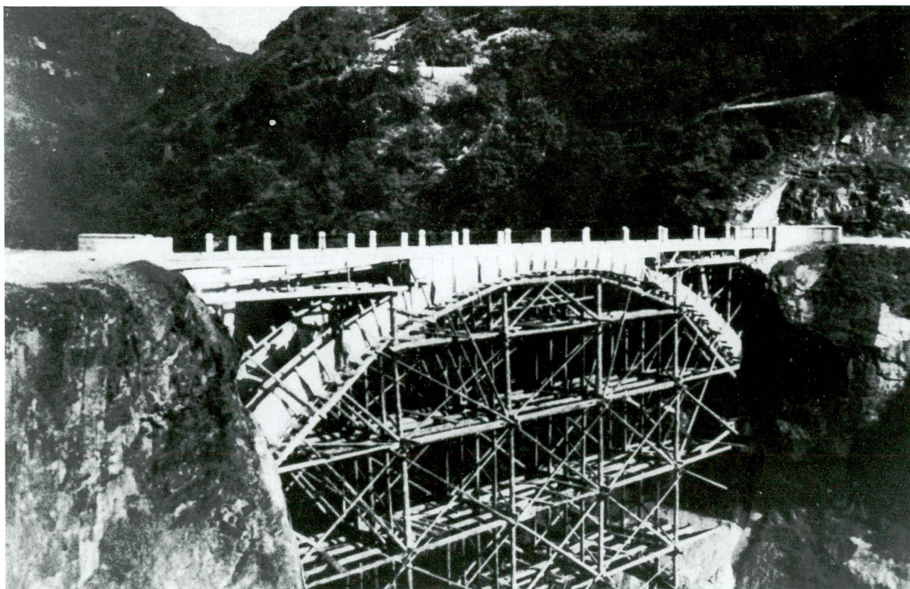
PONTE DEI «TRINGOI» SUL CHIESE NELLA FASE DI COSTRUZIONE (Foto Arturo Ghirardini, Tione).
