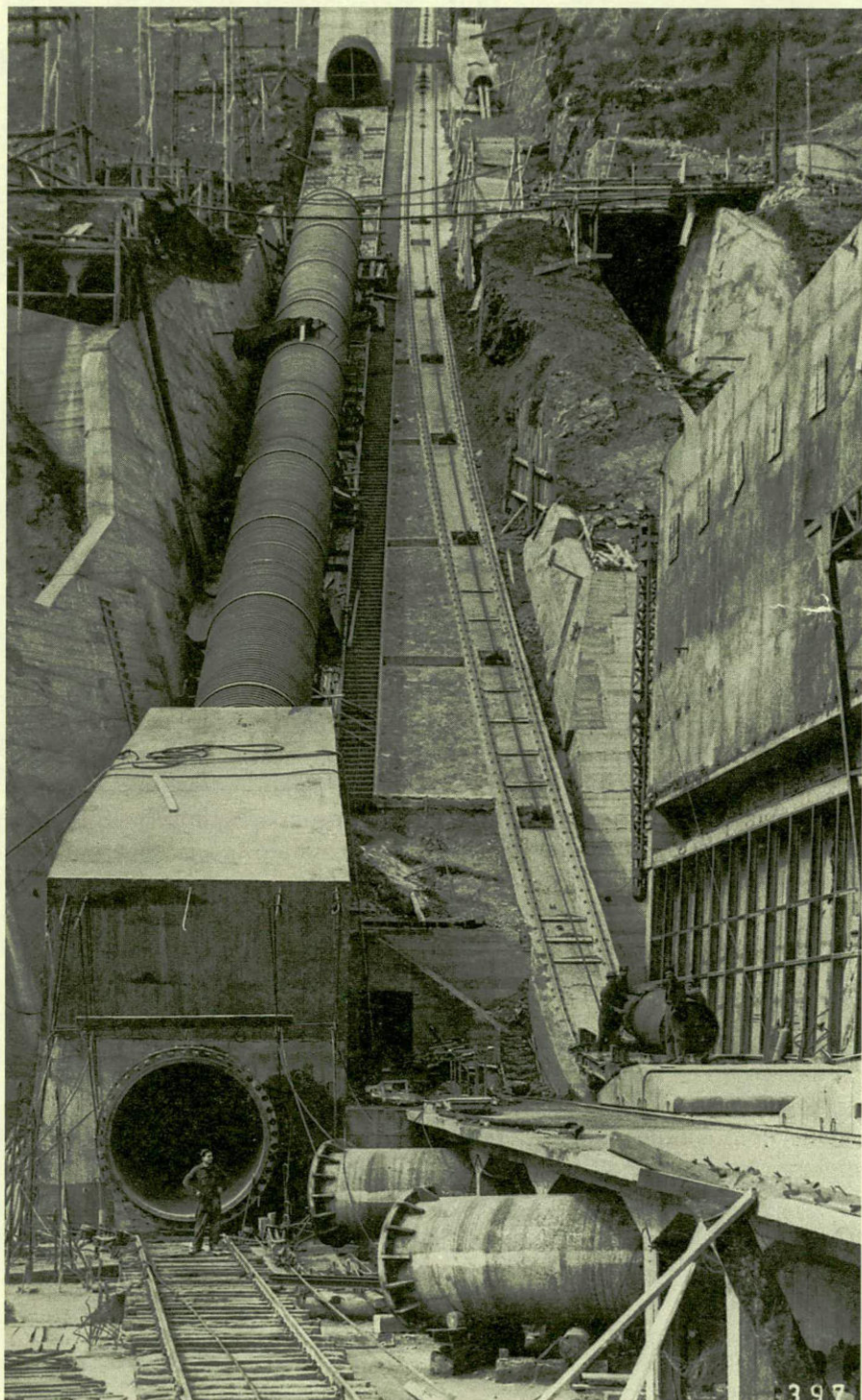
Diga di Boazzo, lavori 1954
