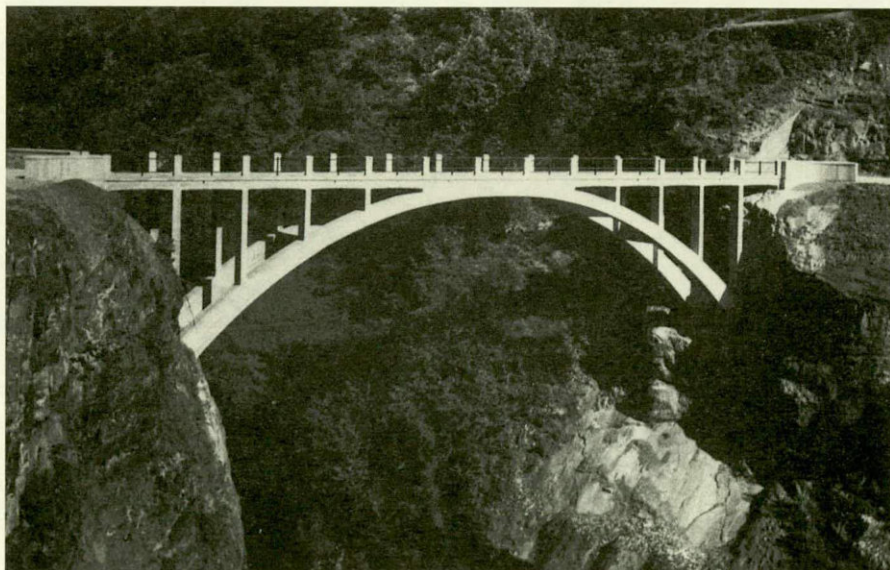
Bersone, ponte dei Tringoi
