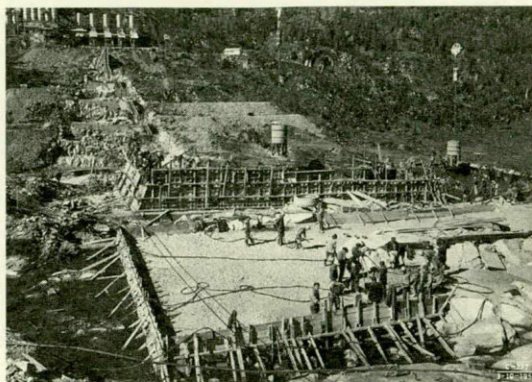
Diga di Bissina
