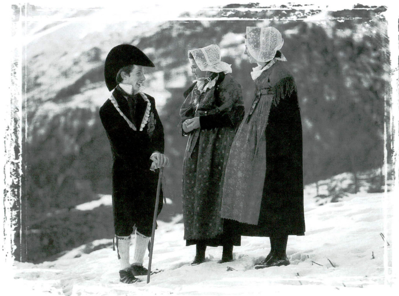
Costumi tipici della Valle Varaita.
